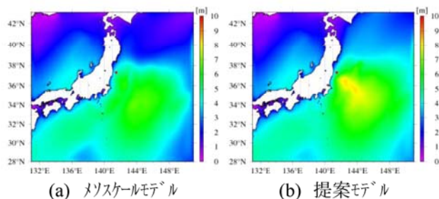
図 10 各モデルによる波浪場 (1995/9/17 18:00)
