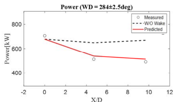
図6 1列風車(WT15-WT12-WT16)の発電量
