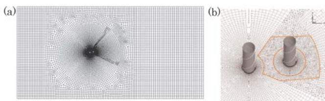
図3 数値解析モデルの(a)解析領域と(b)鳥瞰図
