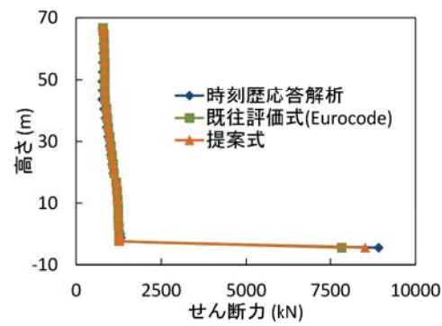
図 3 せん断力の鉛直分布の比較
