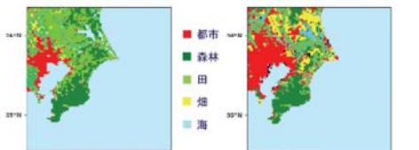
各データベースの土地利用分類の比較
