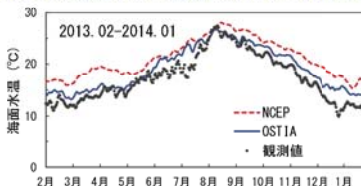
各データベースの海面水温の季節変化
