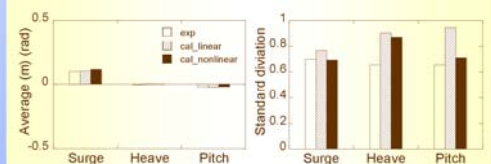
複合外力中における線形モデルと非線形モデルによる 予測値と実験値の比較
