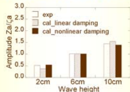
規則波中における動揺の予測値と実験値の比較
