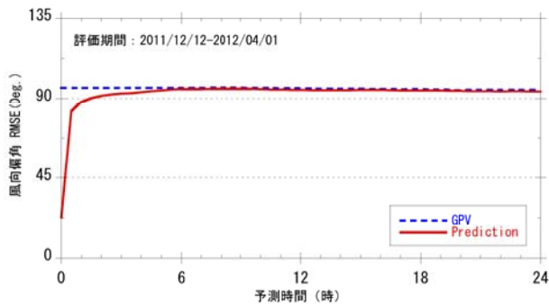
図 3 風向予報誤差の RMSE
