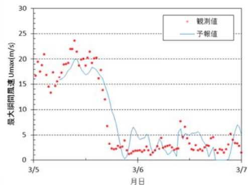
図 5 最大瞬間風速の 6 時間先予報結果
