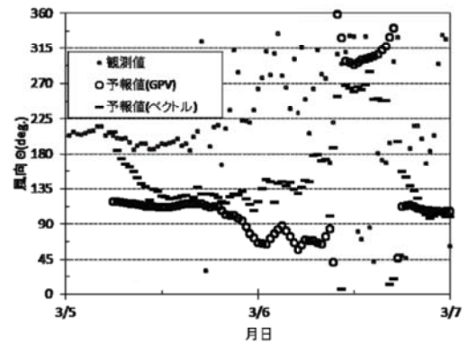
図2 風向予報の例
