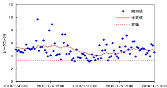
図 4 ピークファクタの観測と推定結果
