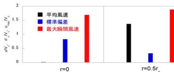
図7 地表面付近( z=0.2r_c )における最大瞬間風速
