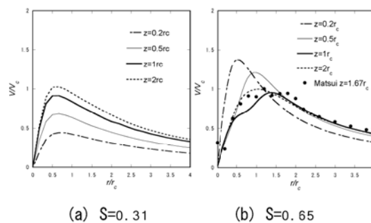
図 3 無次元化円周風速の半径方向分布
