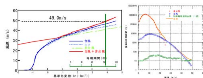
図7 対象海域における風速の再現期間別期待値
