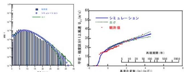
図5 銚子気象台における台風時の風速階級別出現頻度
