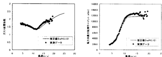
(a) ガスト影響係数 (b) 最大転倒モーメント
