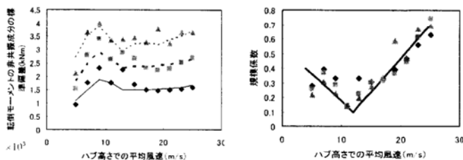
(a) 非共振成分の標準偏差 (b) 規模係数 K
