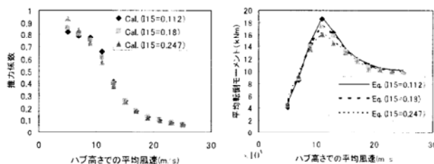
(a)スラスト係数 (b)平均転倒モーメント
