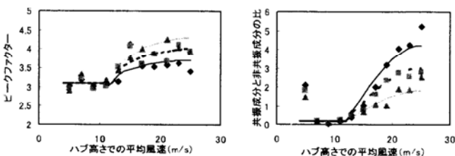
(a) ピークファクター (b) 共振と非共振成分の比
