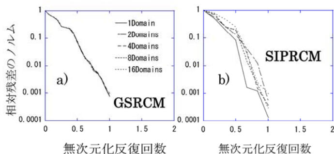
図-5 新しい並列解法による収束の様子
