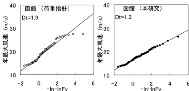
図3 測器補正による年最大風速の極値分布の変化
