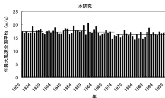
図2 測器補正後の年最大風速の経年変化
