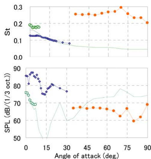
図2 ピーク St と音圧レベル, W/B=3 (実線: \square 20 \times 60\text{mm} の矩形柱)
