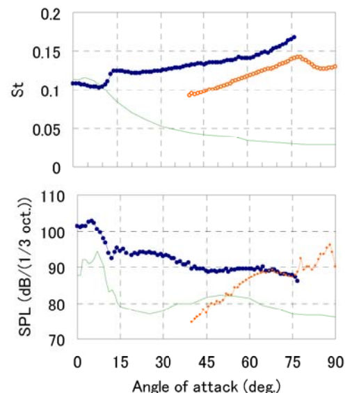
図3 ピーク St と音圧レベル, W/B=5 (実線: \square 10 \times 50\text{mm} の矩形柱)
