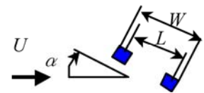
図1 模型配置図
