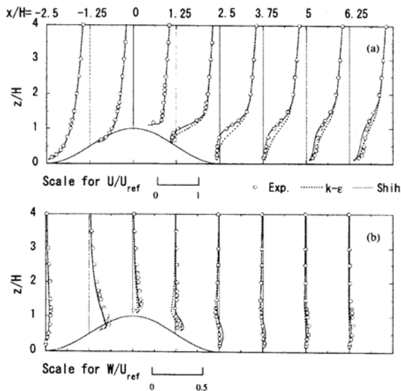
図3 3次元山の中心断面における平均速度成分 U , W の鉛直分布
