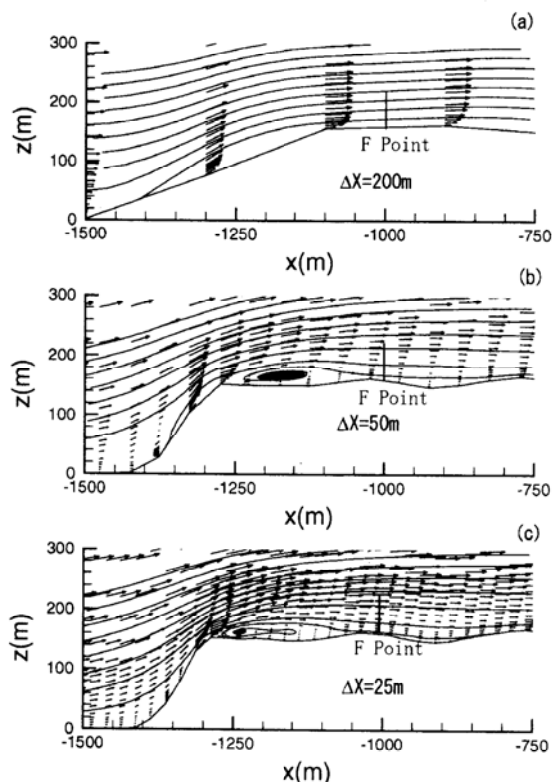
図 9 平均風速のベクトル図
