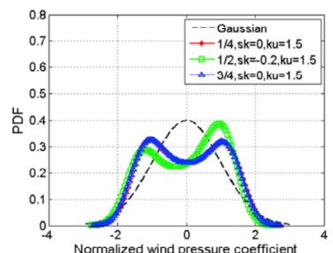
(d) Curved roof ( f_m=50\text{Hz} )
