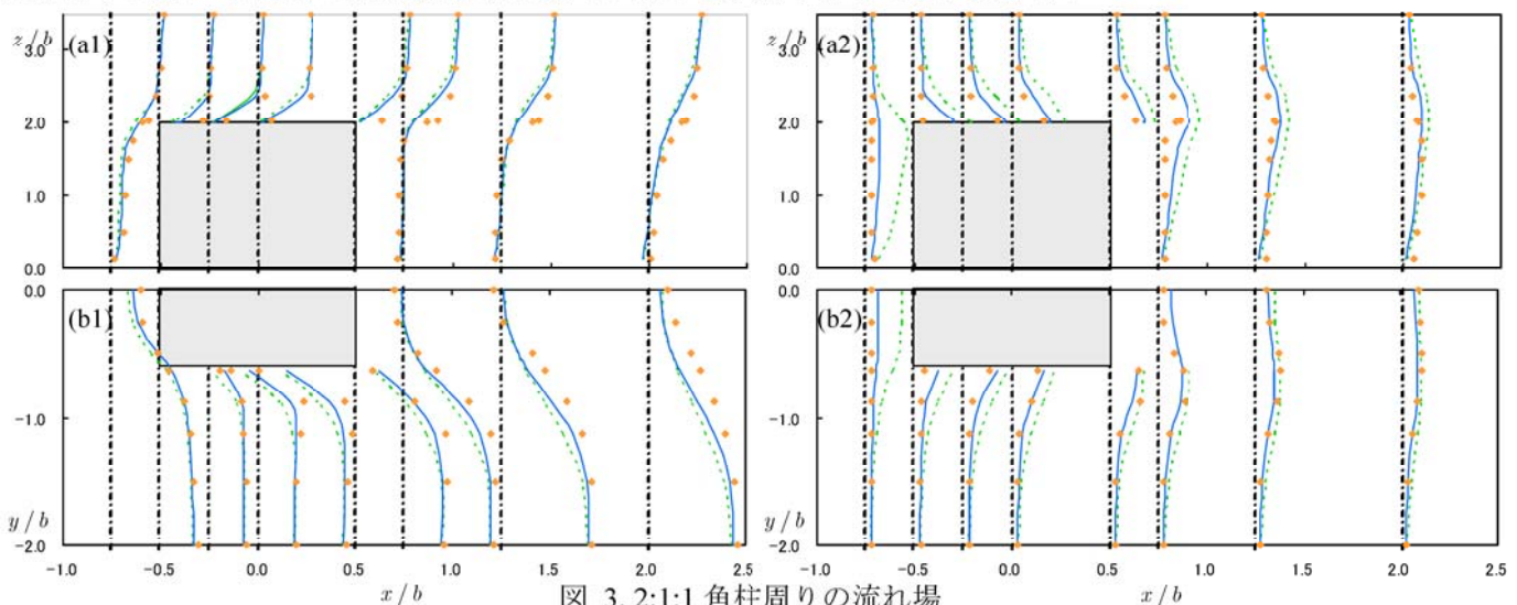
図 3. 2:1:1 角柱周りの流れ場
