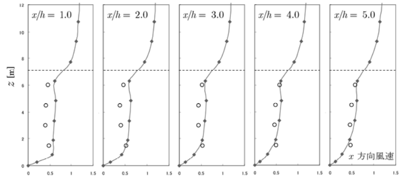
図 2. 樹木背後の流れ場
