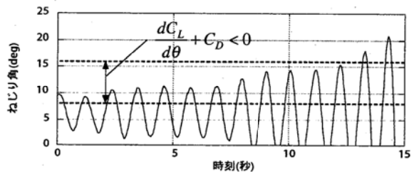
(c) 1-1.00D, 乱流:発生風速12.2m/s, 平均値6.4deg
