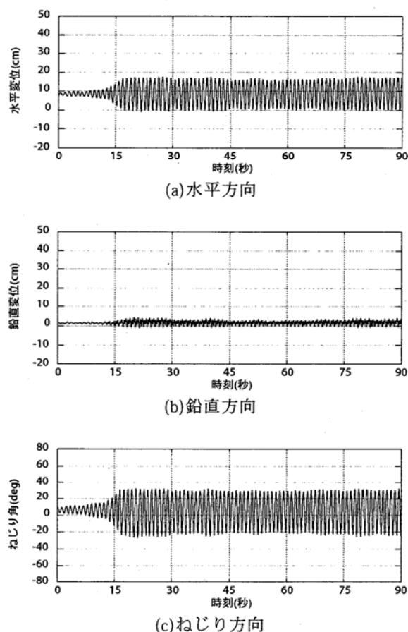
図-16 ギャロッピング発生時変位時刻歴:1-1.00D, 乱流
