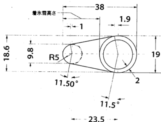
(a)4-1.00D (4本用いる)
