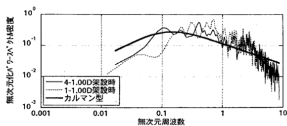
図-18 ギャロッピング発生時の変動風速パワースペクトル密度
