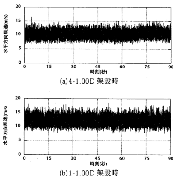
図-17 ギャロッピング発生時の変動風速時刻歴
