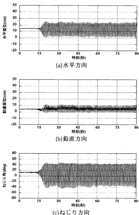
図-15 ギャロッピング発生時変位時刻歴:1-1.00D, 一様流
