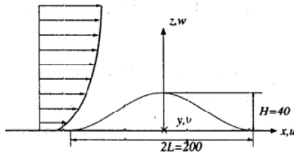
図1 2次元尾根の形状 (平均傾斜角 21.8 度)
