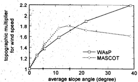
図4 山頂での風速比の傾斜角度による変化
