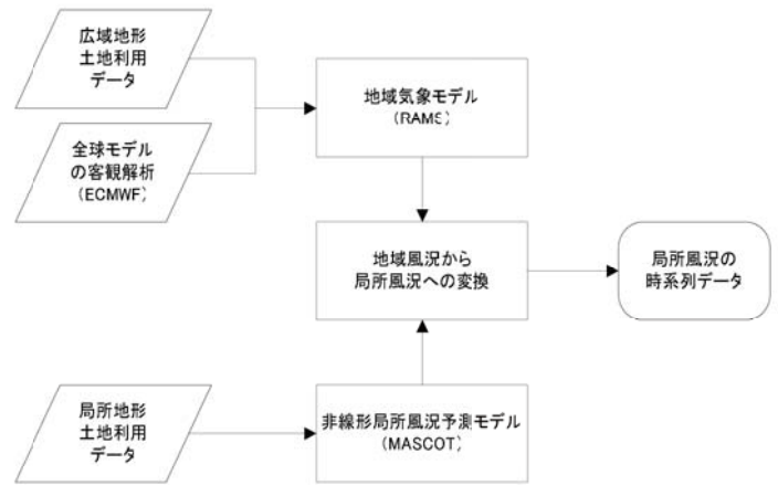
図1 力学統計的局所化手法の流れ
