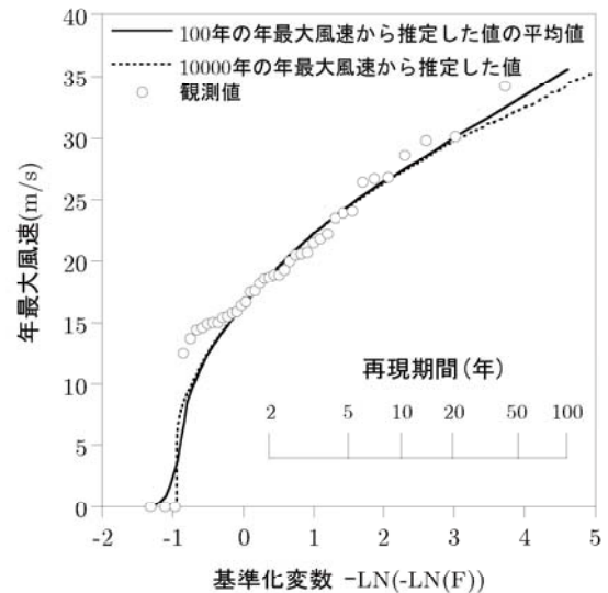
図 9 銚子気象台(粗度区分 II, h=10m)における台風時の年最大風速の確率分布
