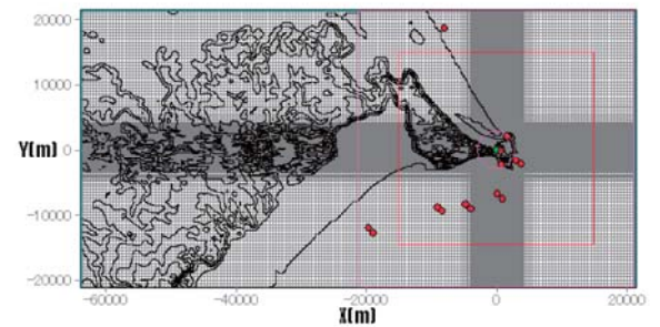
図 4 局所風況予測モデルの解析領域
