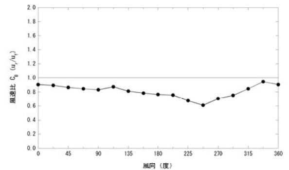
図 5 銚子気象台における風速割増係数
