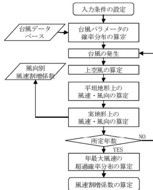
図2 台風シミュレーションの流れ
