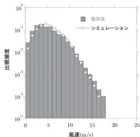
図 7 銚子気象台における風速階級別出現頻度分布
