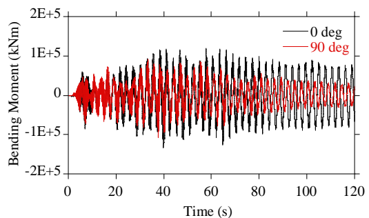
図5 停止時のタワー基部曲げモーメント時刻歴
