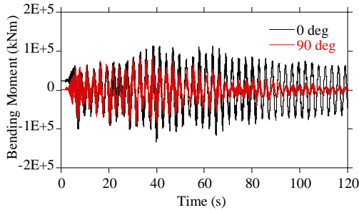
図6 緊急停止時のタワー基部曲げモーメント時刻歴
