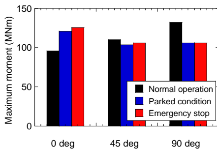
図7 タワー基部曲げモーメント最大値のまとめ
