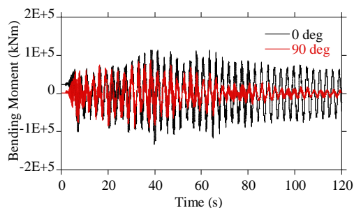
図 5 緊急停止時のタワー基部曲げモーメントの時刻歴
