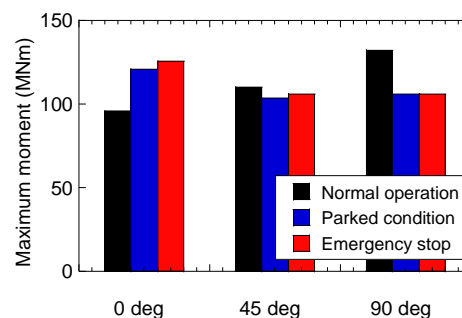
図 6 タワー基部曲げモーメント最大値のまとめ
