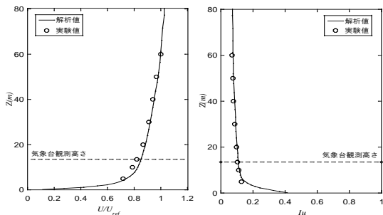
図 4 平坦地形上の無次元風速と乱れ強さの鉛直分布
