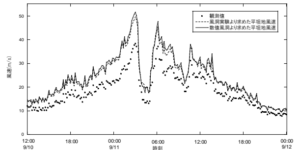
図 7 気象台高さにおける観測値と平坦地形上風速
