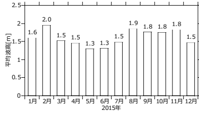
(a)月別平均波高
