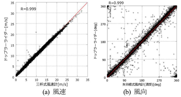
Fig.6 タワー観測値とドップラーライダーとの比較
