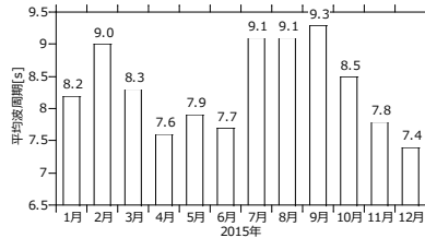
(b)月別平均波周期
