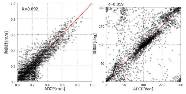
(a) 流速 (b) 流向 Fig.9 海象計と ADCP との比較
