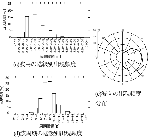
Fig.11 波浪データの統計分析結果
