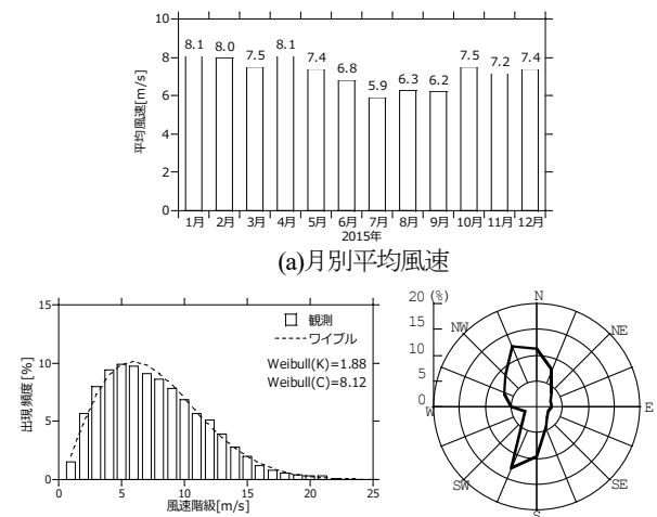
(a) 月別平均風速 (b) 風速の階級別出現頻度 (c) 風向の出現頻度分布
