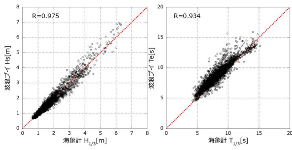
(a) 波高 (b) 波周期 Fig.8 波浪ブイと海象計との比較
