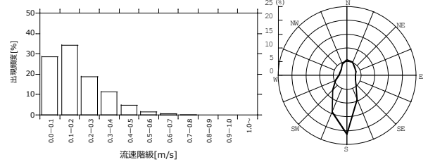
(b)流速の階級別出現頻度
