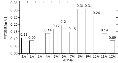
(a)月別平均流速
