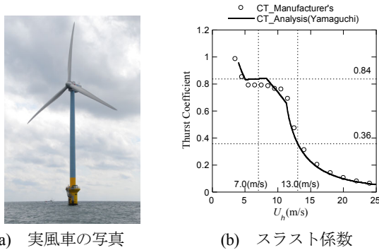
図3 銚子沖 2400kW 洋上風車
