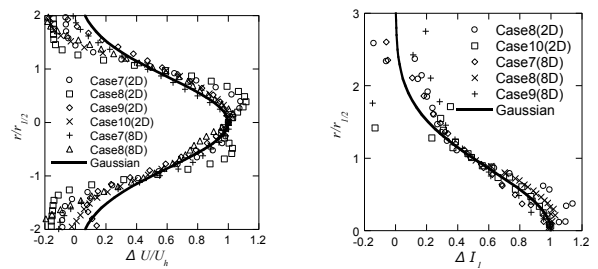
(a) 風速欠損 (b) 乱流増分
