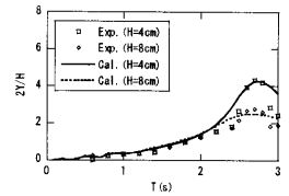
図 3 サージの周波数応答関数
