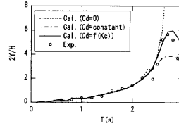
図 2 抗力係数がサージに与える影響
