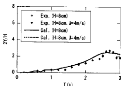
(b) 暴風時
