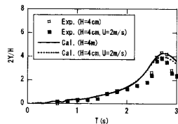
(a) 発電時
