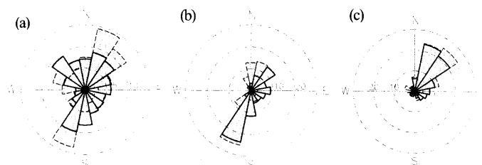
図4 銚子気象台における風況図 (a)年間、(b)6月、(c)10月
