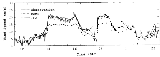
図3 竜飛岬灯台での10分平均風速の時系列(1月)
