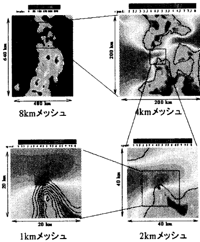
図2 地域気象モデルの計算領域
