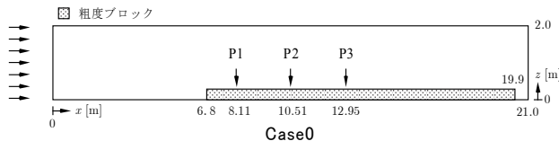
図-13 実験概要と気流計測点の位置
