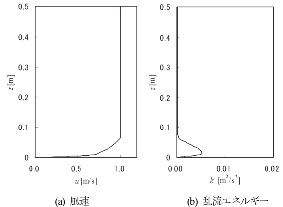
図-15 キャノピー層解析に用いた流入風
