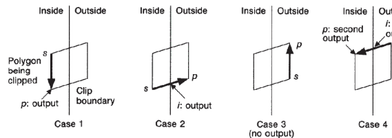
図-9 Sutherland and Hodgman 法のクリッピングウィンドウ境界における内外の判定と境界上の交点の処理 42)
