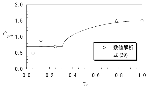
図-5 モデル定数 C_{pe2} と占有率 \gamma_o の関係
