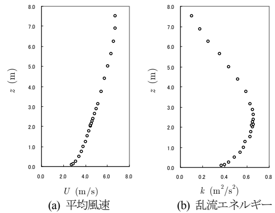
図-19 流入風
