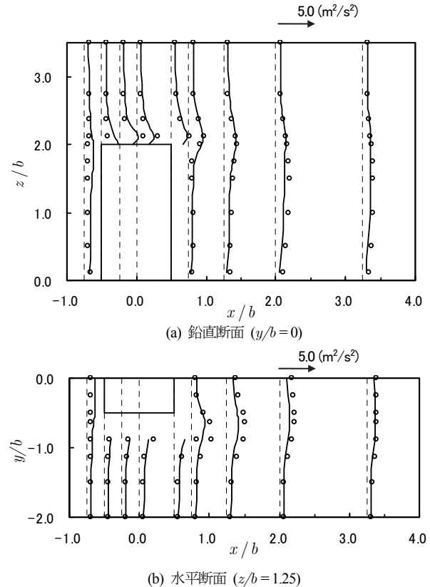
図-21 角柱周りの乱流エネルギーの予測値と実験値 45) との比較
