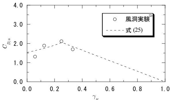
図-1 抗力係数 C_{D,u} の占有率 \gamma_u による変化
