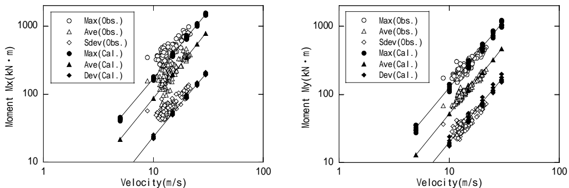
図 9 風車タワー基部における X 方向と Y 方向の曲げモーメントの風速による変化
