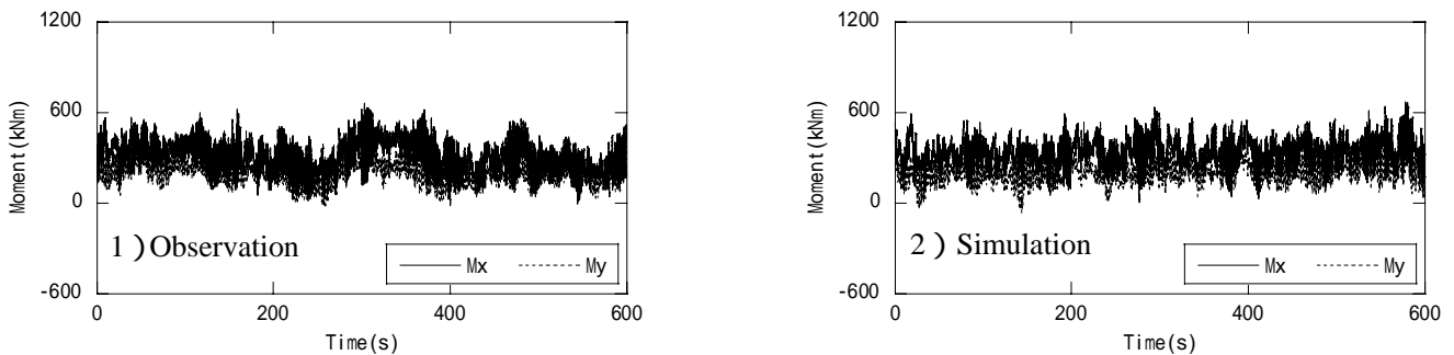
図 8 風車タワー基部における曲げモーメントの時刻歴の観測結果と予測結果との比較
