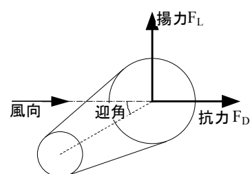
図 5 迎角と空気力の定義
