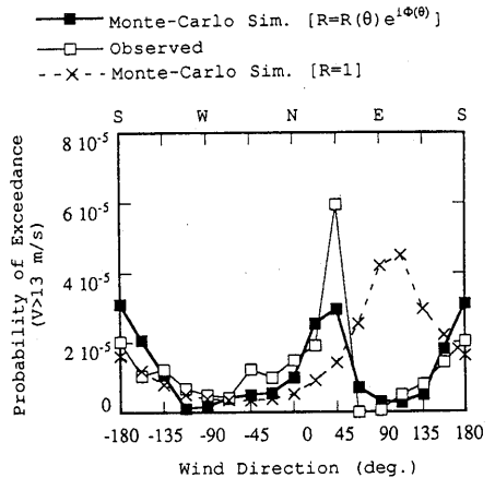
図7 大阪における風向別超過確率
