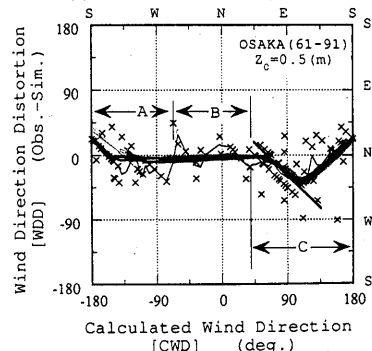
(b) 風向偏差 \Phi
