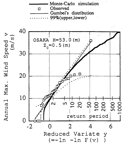
図6 大阪における年最大風速の分布
