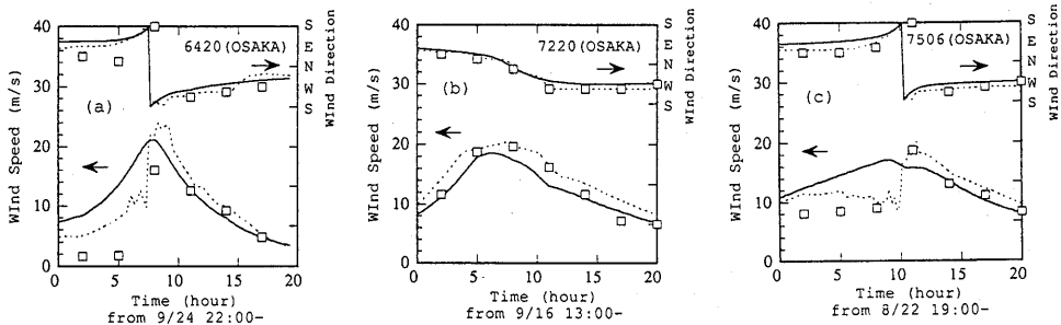
図1 大阪における台風のシミュレーション結果
