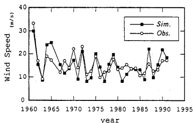
図4 台風による年最大風速(時系列)
