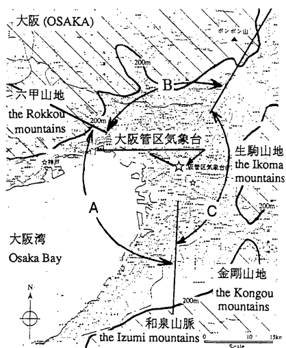
図3 大阪平野における観測点(気象台)位置と周囲の地形の関係
