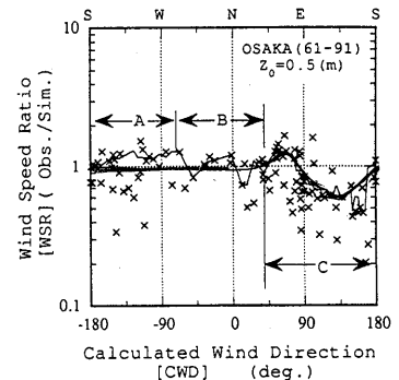
(a) 風速比 R
