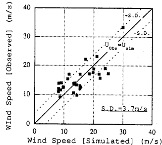
図5 台風による年最大風速(観測値と計算値の比較)
