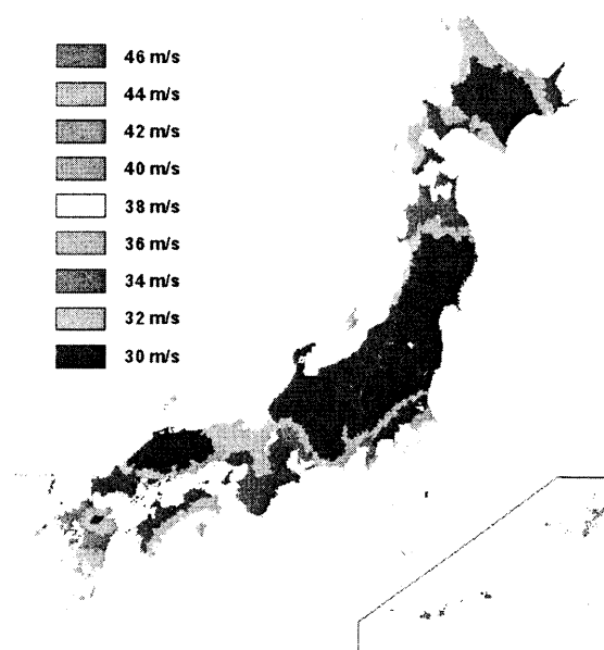
図-3 設計基準風速の分布 8)
